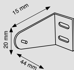
Fixeersteun
