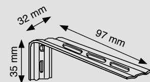
Voorsprongsteun 70 mm
